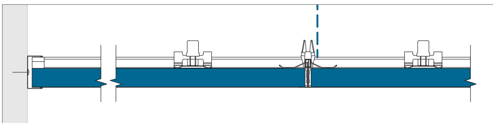
Randafwerking met hoekrandprofiel en wandveer (stootvastheid 3A, 25 mm plafondtegel).
